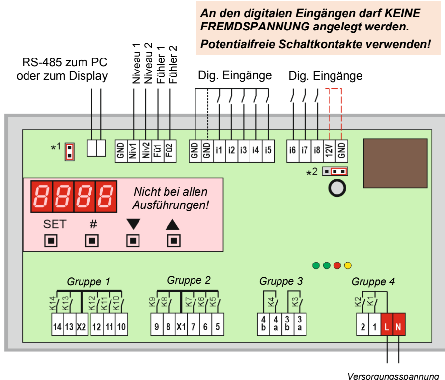
Jumper *1 zum Abschluss Schnittstelle
