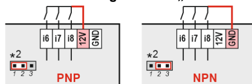
Jumper *2 zur Umschaltung Polarität „i6 – i8“
